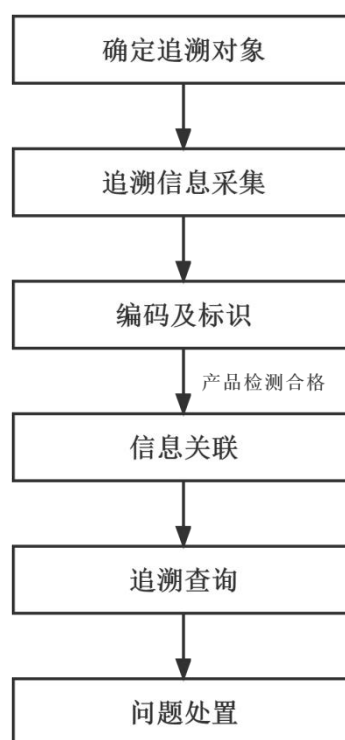
图 1 追溯流程图
