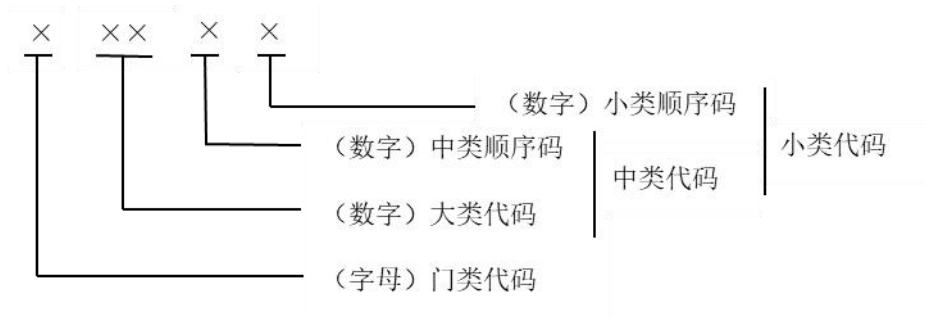
图 1 代码结构图
