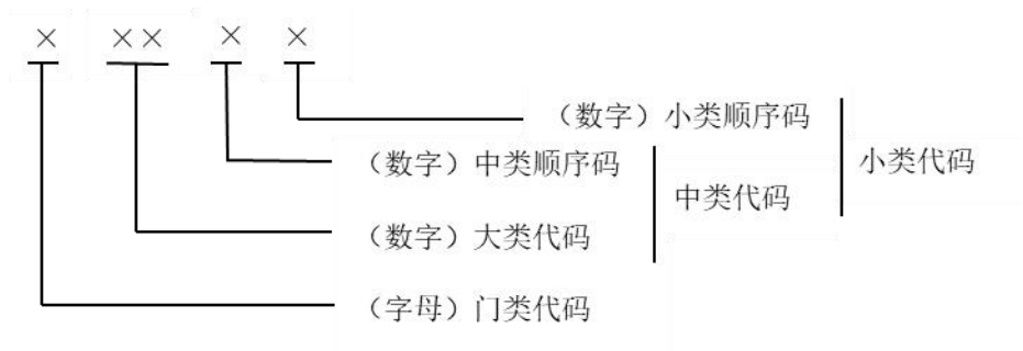
图 1 代码结构图
